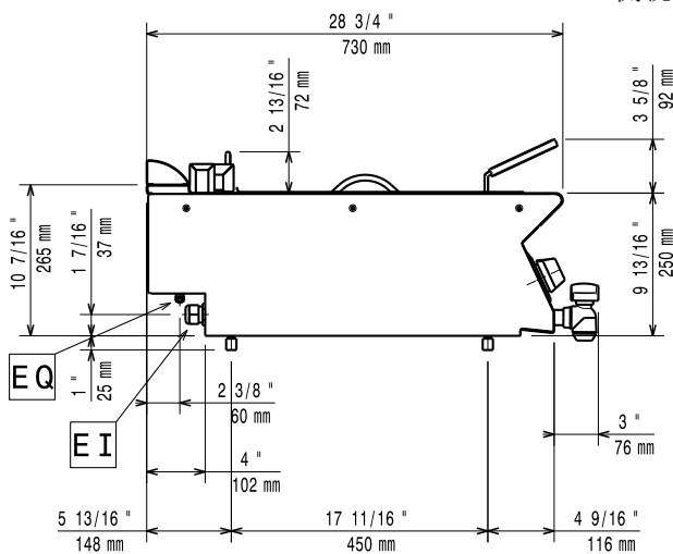
侧视
